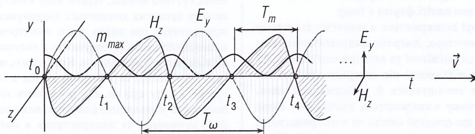
Рис. 2. Представлення часового поширення електромагнітних хвиль
